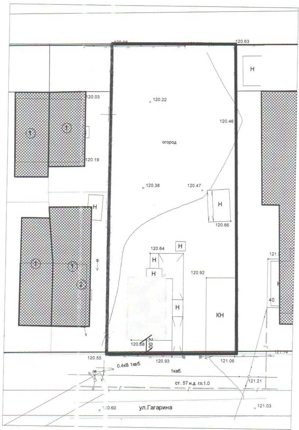
Чертеж планировки территории с отображением красных линий, линий регулирования застройки, осей улиц, линий дорог и проездов
